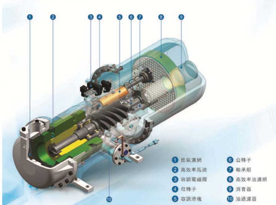
剖面圖說明
